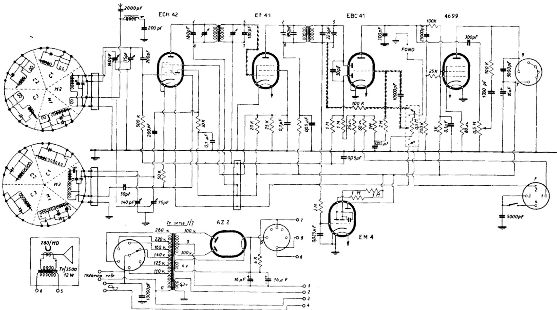
PEBA RADIO (Pertusati) - Mod. ME/505 W 12. Gamme d'onda in metri: M1 320-580, M2 190-320, C1 34-54, C2 21-34 e C3 12,5-21. Media frequenza 467 kc/s. Potenza d'uscita 4,5 watt. Consumo 70 watt.
